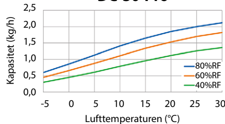
DC-30 T16
