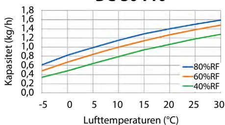
DC-30 T10
